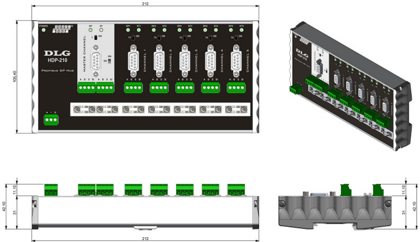
Figura 2 - Dimensionamento para montagem (cotas em milímetros)
