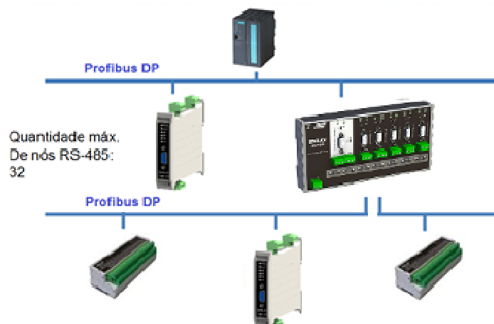
Figura 1 - Aplicação do HDP-210.
